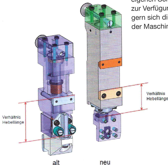
Bild 2: Die neuen verdrehgesicherten Steinführungen mit integriertem Wegmesssystem (re.) haben ein optimiertes Hebelverhältnis zwischen Steinaufnahme und Kontaktzone. Dadurch reduzieren sich die Querkräfte, folglich der Verschleiß an Kolbenstange und Führungsbuchse. Die neuen Steinführungen sind auf Maschinen der älteren Generation adaptierbar
